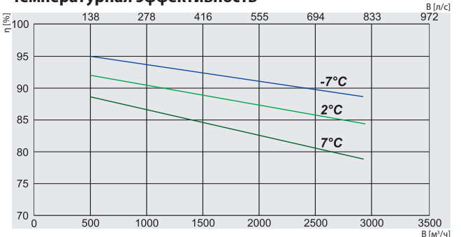
Температурная эффективность
