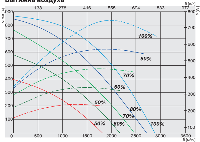
Удельная мощность вентилятора
